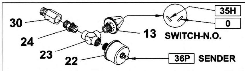
HRMTR ENG OIL PRESS SW-N.O. & OIL PRESS SENDER
